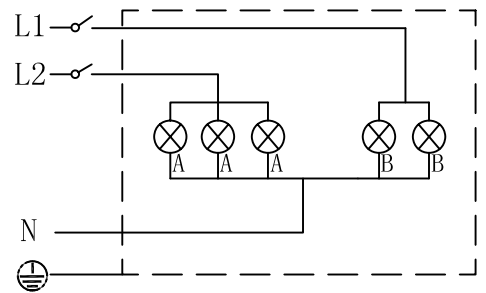
CIRCUIT SCHEMATIC принципиальная (электрическая) схема
