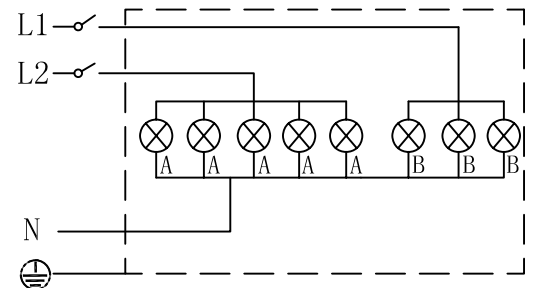
CIRCUIT SCHEMATIC принципиальная (электрическая) схема
