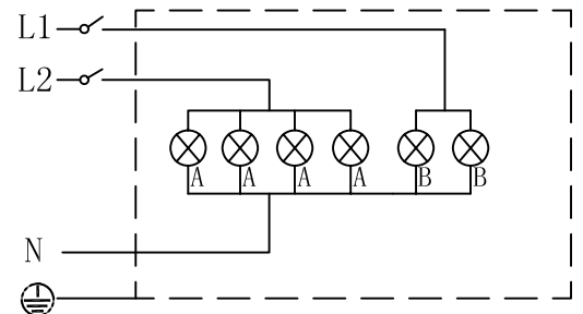
CIRCUIT SCHEMATIC принципиальная (электрическая) схема
