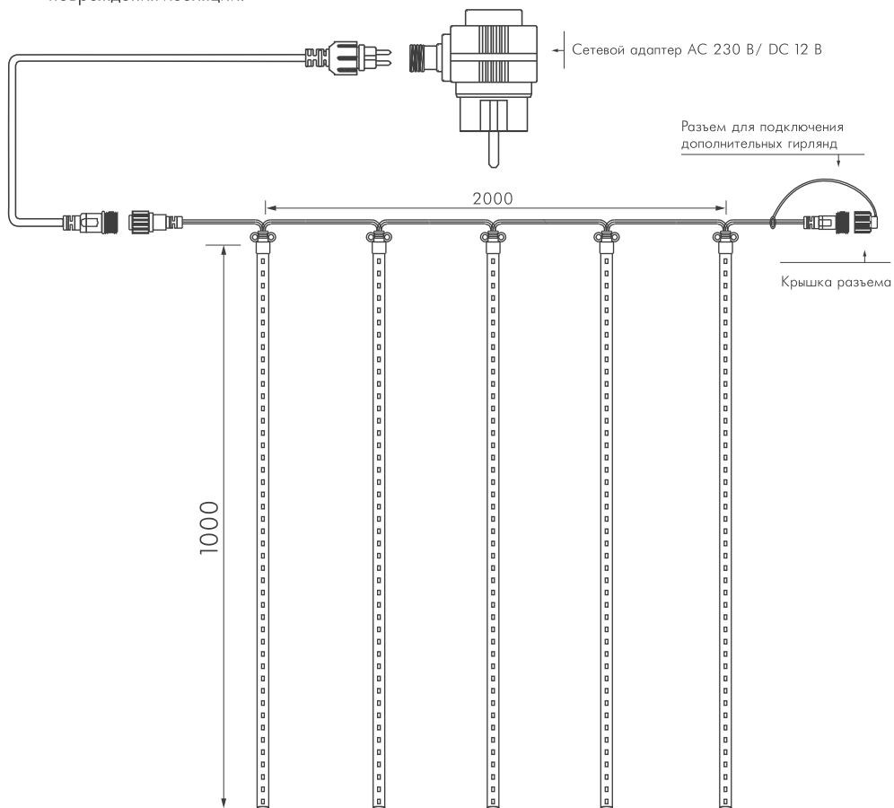
Рисунок 1. Схема подключения.
