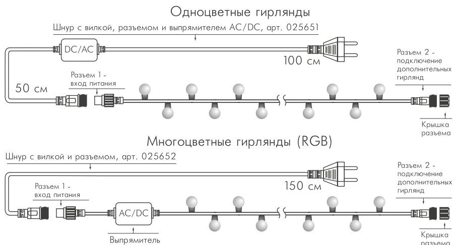
Рисунок 1. Схемы подключения.
