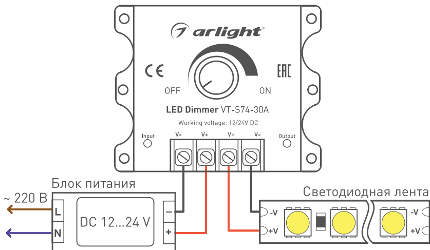
Рис. 1. Схема подключения диммера.
