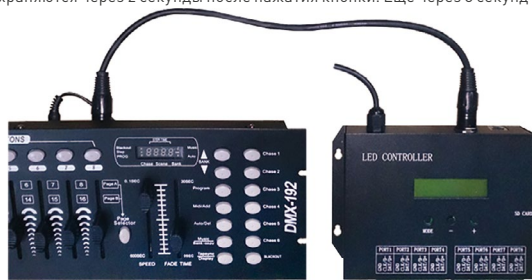
Рис. 4. Подключение DMX-консоли для управления контроллером.
