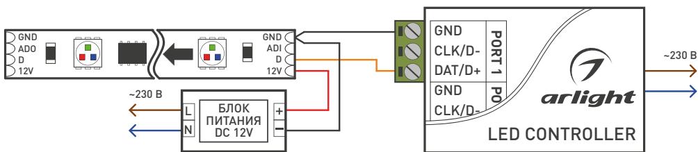
Рис. 2. Подключение светодиодной ленты или модулей с интерфейсом SPI.
