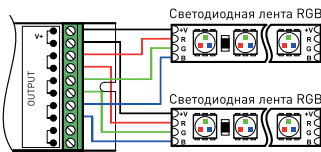
Схема 2. Подключение светодиодной ленты RGB.
